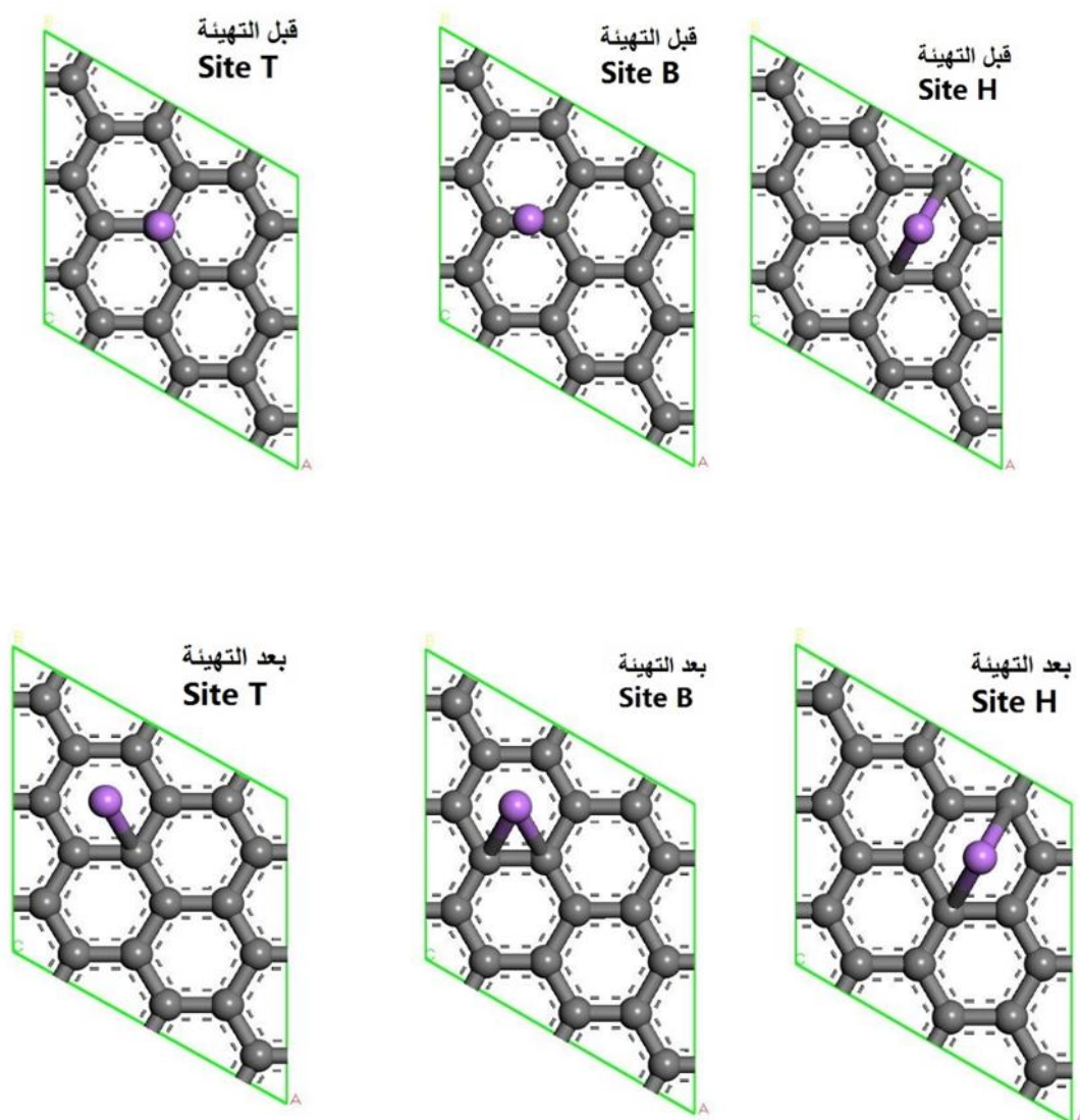
شكل 3: مواقع الامتزاز قبل وبعد تهيئة ذرة الليثيوم (اللون البنفسجي) على سطح الغرافين (اللون الرصاصي).
