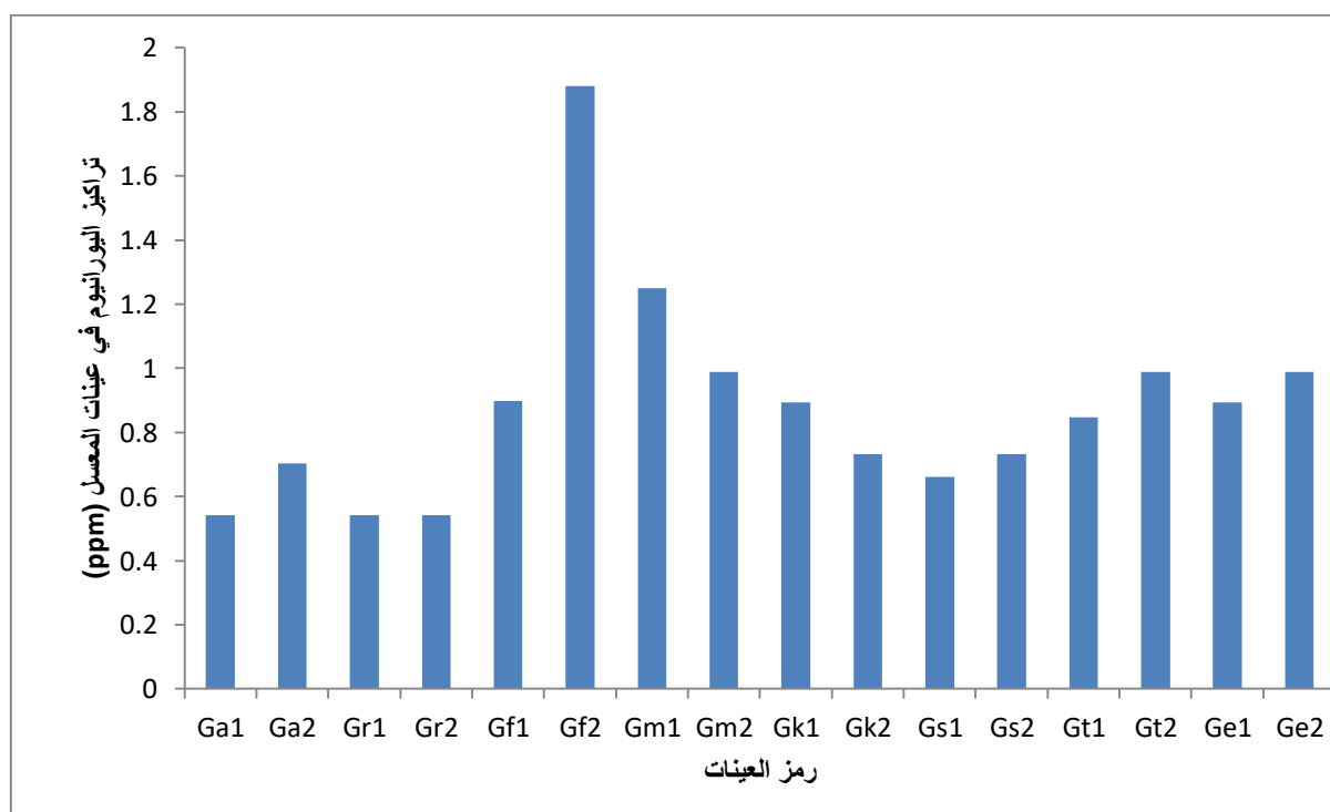
شكل 8: تراكيز اليورانيوم (ppm) في عينات المعسل.
