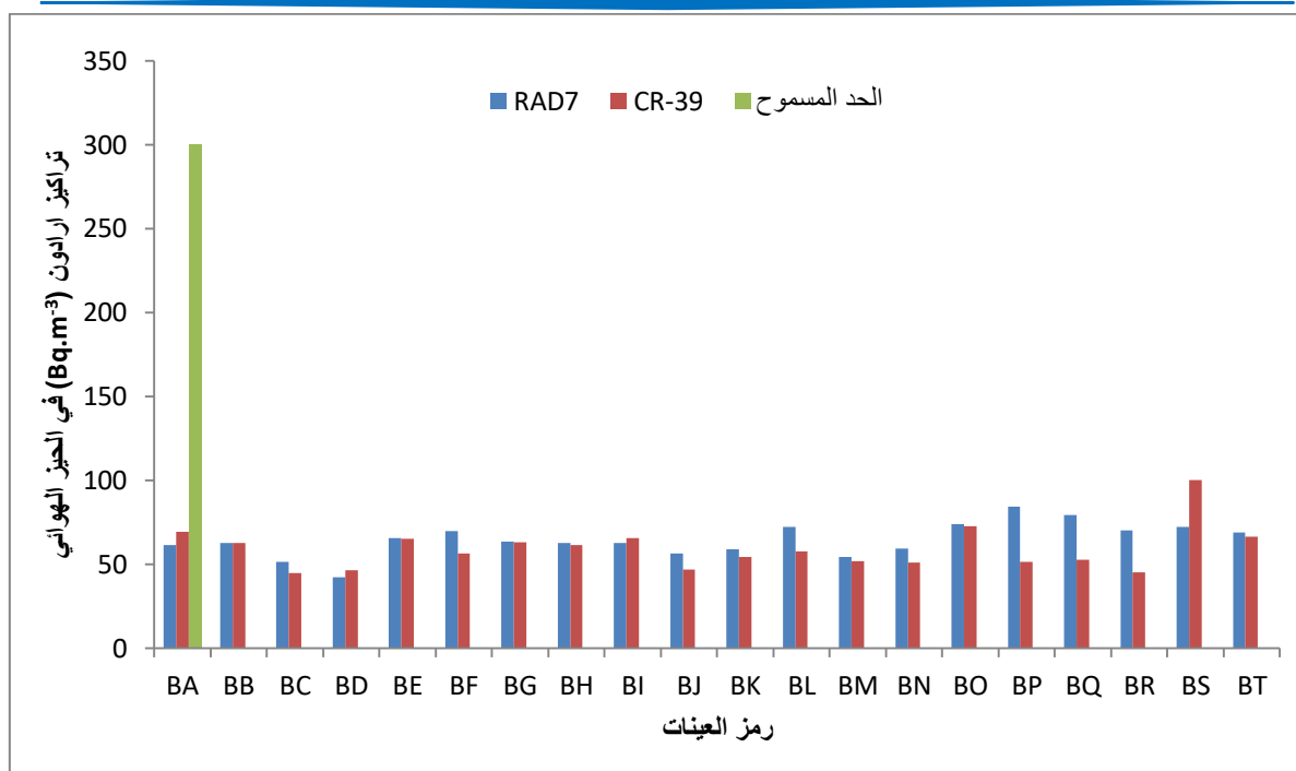
شكل 3: تراكيز الرادون في الحيز الهوائي داخل الاسطوانة المقاسة بواسطة كاشف CR-39 و RAD7 في عينات تبغ السكاثر والحد المسموح به [1].
