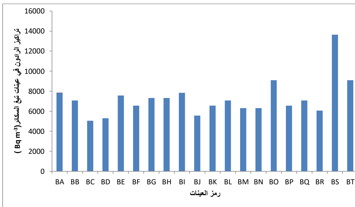
شكل 4: تراكيز الرادون في عينات تبغ السكاثر.
