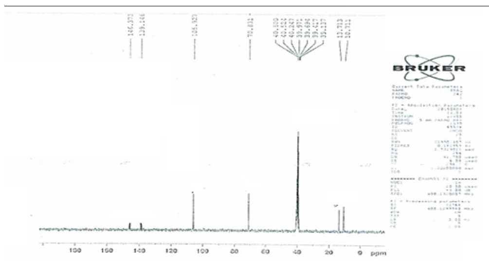
الشكل (3) طيف الرنين النووي المغناطيسي ^1\text{H-NMR} للمركب (H 4 )
