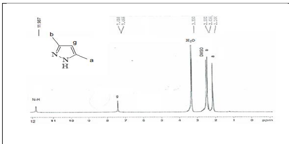
الشكل (1) طيف الرنين النووي المغناطيسي ^1\text{H} -NMR للمركب (H 1 )
