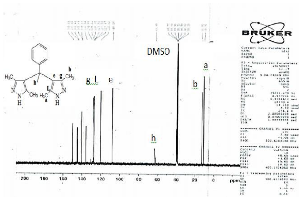
الشكل (6) طيف الرنين النووي المغناطيسي 13 C-NMR للمركب (H 5 )
