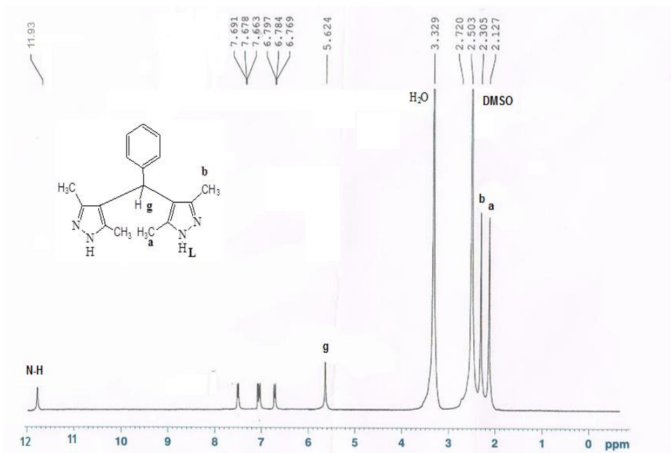
الشكل (5) طيف الرنين النووي المغناطيسي 1 H-NMR للمركب (H 5 )
