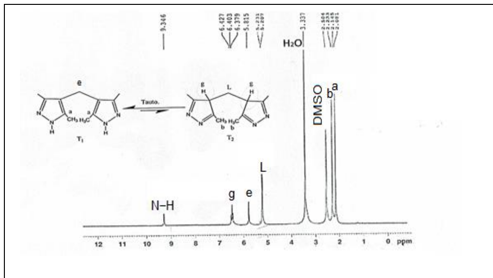
الشكل (3) طيف الرنين النووي المغناطيسي ^1\text{H-NMR} للمركب (H 4 )
