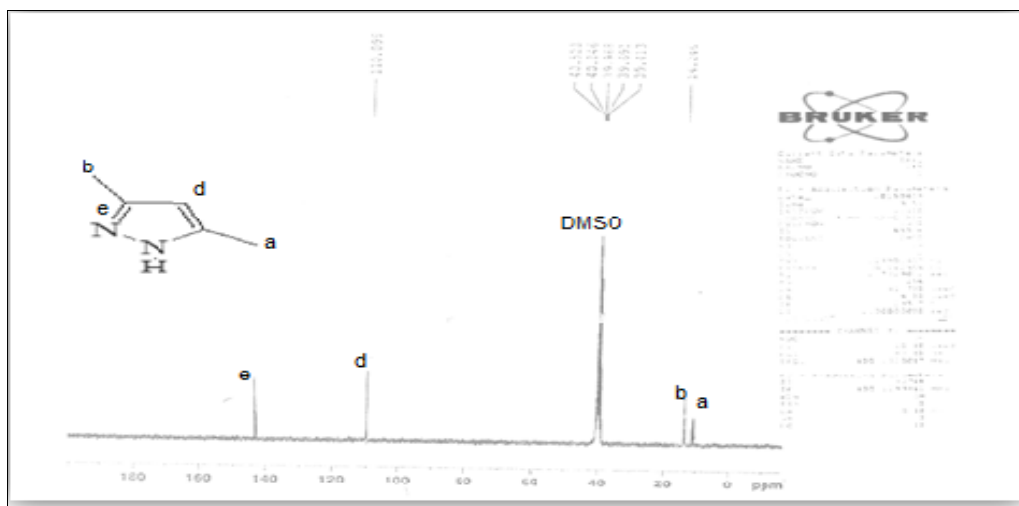
الشكل (2) طيف الرنين النووي المغناطيسي ^{13}\text{C} -NMR للمركب (H 1 )
